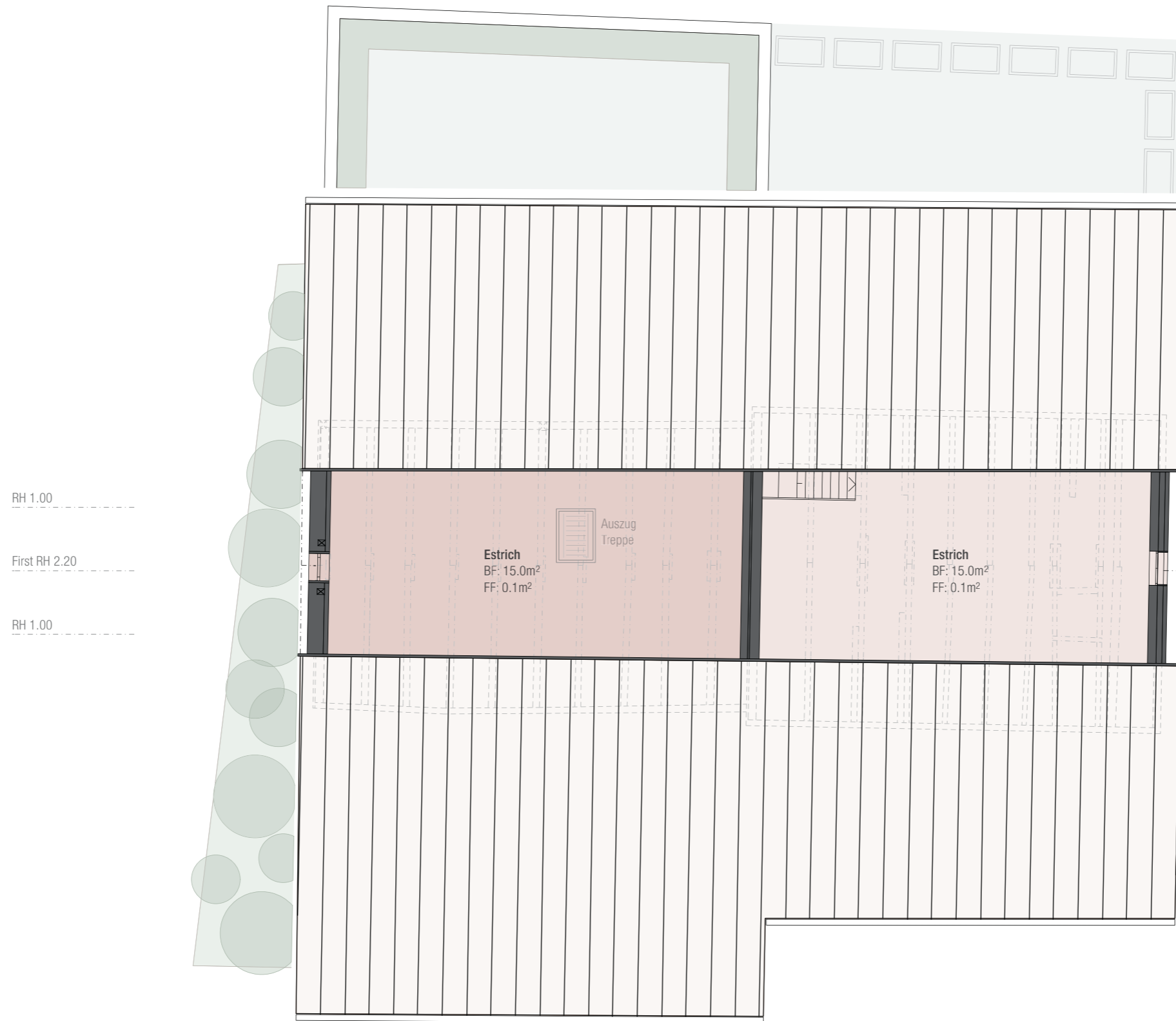
Haus A | Grundriss 2.Dachgeschoss | M 1:100
